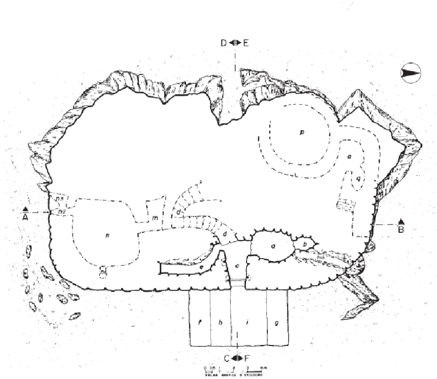
Fig. 1 - Nuraga Albucciu, planimetría de la planta baja (de ANTONA RUJU, CERUTI 1992, fig. 12).
