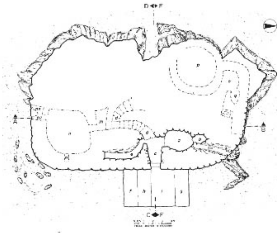
Fig. 1 - Nuraga Albucciu, planimetría de la planta baja (de Antona Ruju, Ferrarese Ceruti 1992, fig. 12).
