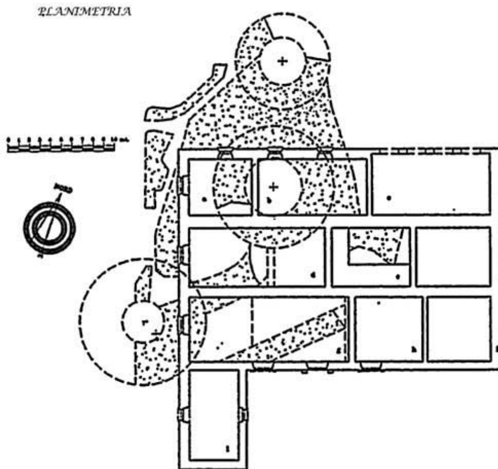
Fig. 1 - Planimetría de los restos arqueológicos del nuraga Su Nuraxi 'e Cresia (de http://barumini.altervista.org/foto/planimetria-copia.jpg ).
