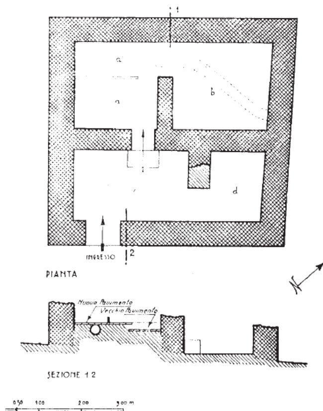
Fig. 2 - Planimetría y sección de la casa romana de Marfudi (de Lilliu 1946, fig. 6, pág. 190).
