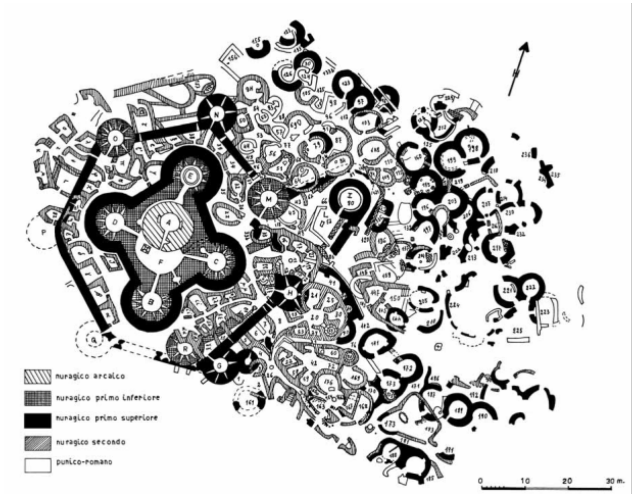
Fig. 1 - Planimetría del yacimiento de Su Nuraxi, nuraga y aldea (de Lilliu 1962, lámina LVI.1, pág. 328).
