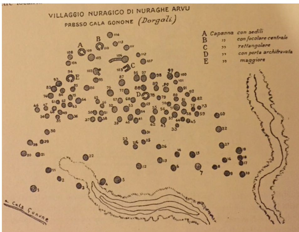
Fig. 3 - Planimetría de la aldea nurágica del nuraga Arvu (de TARAMELLI 1933, fig. 24, pág. 460).
