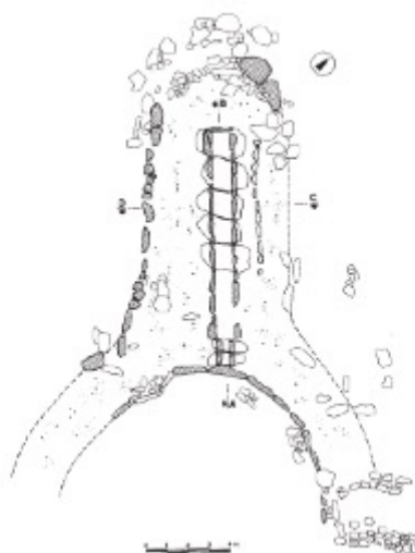
Fig. 1 - Planimetría de la tumba de los gigantes de Thomes (de MORAVETTI 1998, fig. 62, pág. 76).
