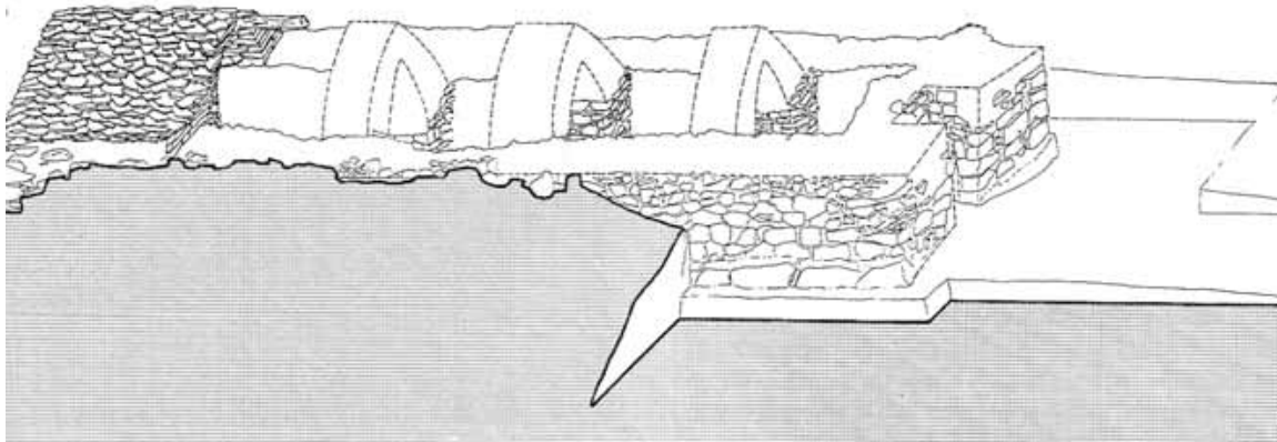
Fig. 3 - Reconstrucción hipotética de la cubierta del megaron 1 (de FADDA 2012, pág. 13, fig. 14).
