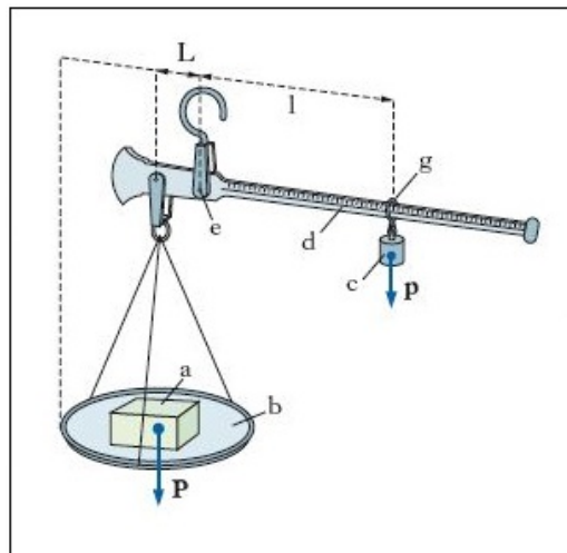
Fig. 3 - El sistema de pesaje de la romana (de http://www.treccani.it/enciclopedia/stadera/ ).
