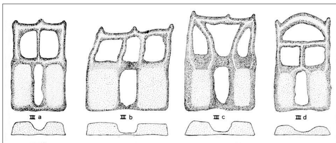
Fig. 3 - Diseño de lingotes de estaño recuperado de los restos de Port Vendres II (de COLLS ET ALII 1975, p. 64, fig. 2).
