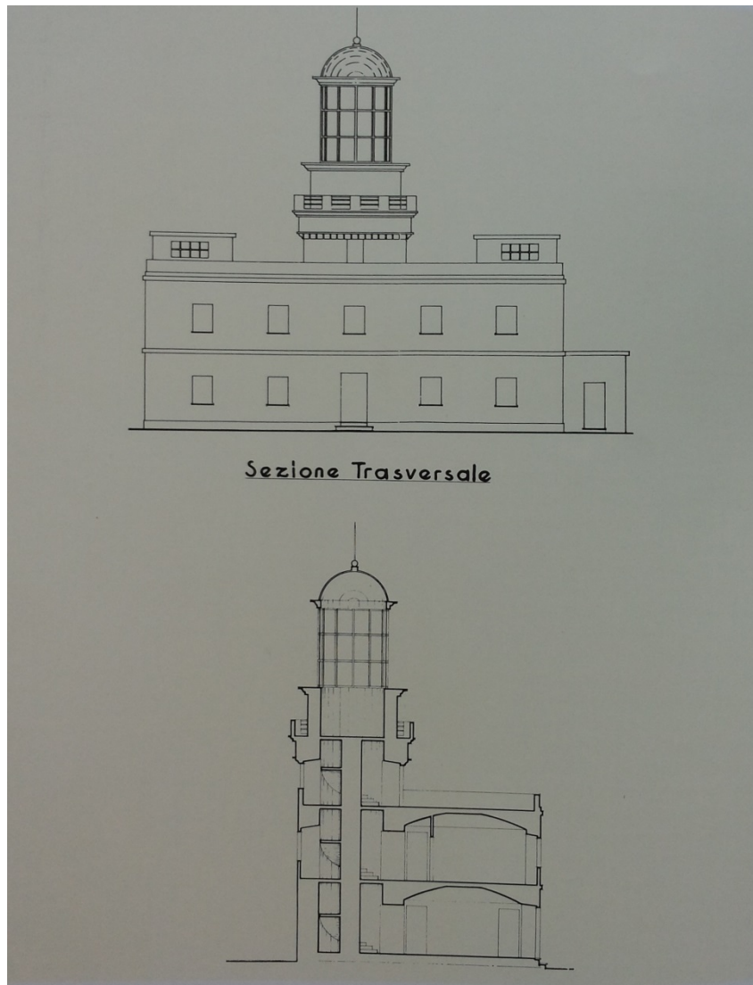
Fig. 4 - Lado principal y sección transversal del faro (de CALANCA 2006, pág. 106).
