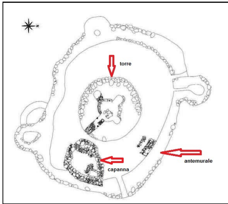
Fig. 4 - Planimetría del nuraga S'Ortali 'e su Monte: se ve el antemuro con torres y las cabañas construidas dentro del antemuro (de Fadda 2012, fig. 43, pág. 33; reelaborado por M. G. Arru).
