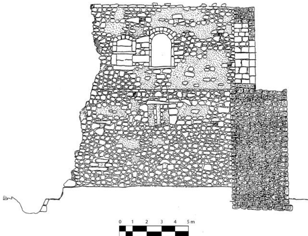
Fig. 4 - Luogosanto, Palazzo di Baldu: interior del lado oeste del Palazzo di Baldu (elaborac. gráfica de A. M. Azara).
