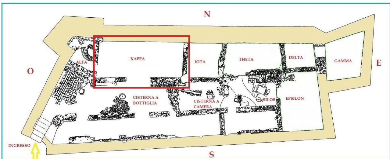
Fig. 1 - El ambiente kappa (reelaborado por M. G. Arru de SPANU 2003, pág. 58).
