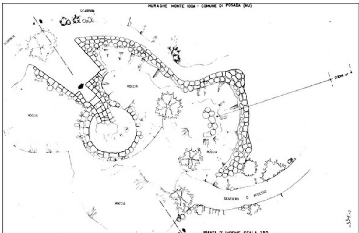
Fig. 3 - Planimetría del nuraga de Monte Idda (de FADDA, 1984 fig. 1).
