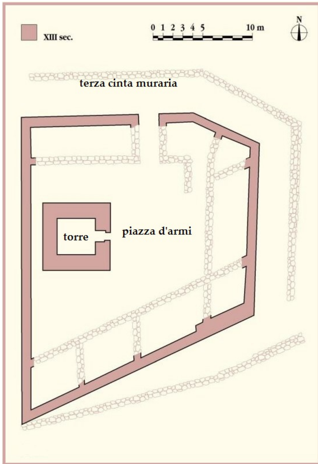
Fig. 5 - Planta del Castillo della Fava, Posada (de CORONEO 1993, ficha 177, pág. 295)
