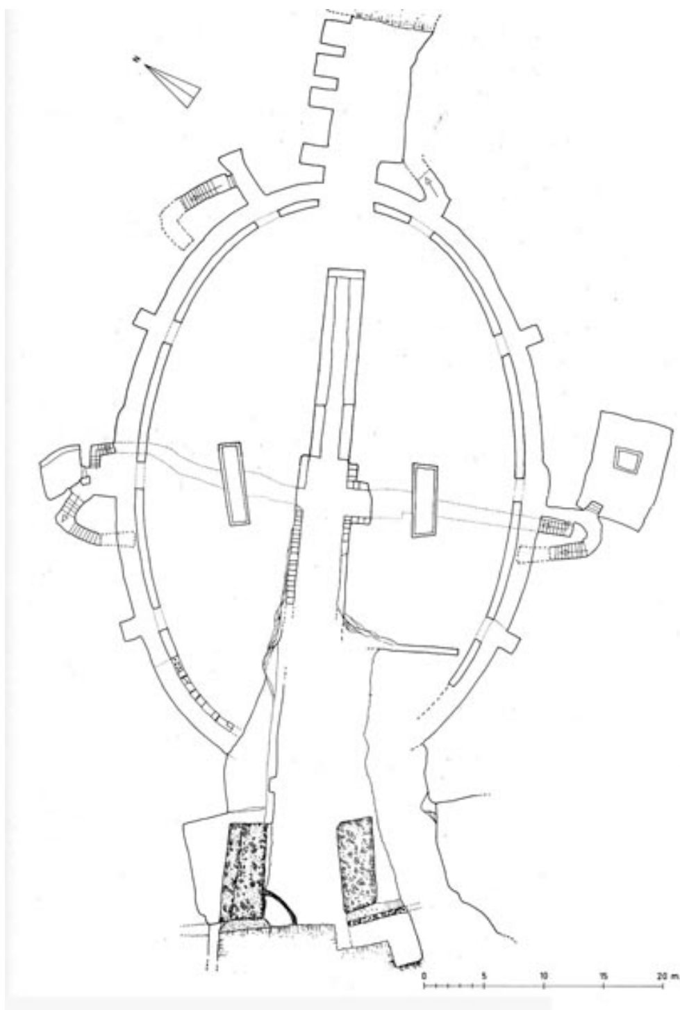
Fig. 4 - Planta del anfiteatro romano de Cagliari (de Pala 1994, pág. 147)
