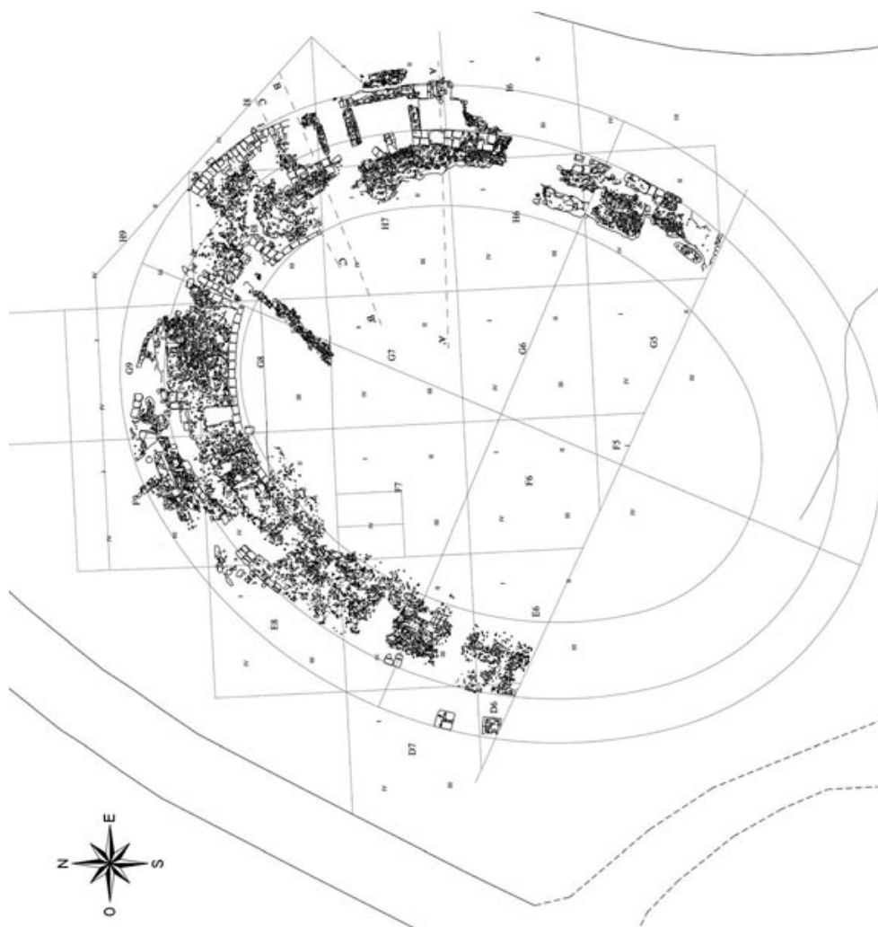
Fig. 2 - Anfiteatro romano de Fordongianus: planimetría en relieve (de Bacco y otros 2010, pág. 1396).
