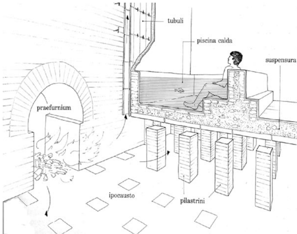
Fig. 2 - Sistema de calentamiento de los ambientes: el aire proveniente del horno entraba bajo el suelo sostenido por suspensurae y, a través de los tubuli perforados dentro de las paredes, creaba un aislante caliente del espacio (de Adam 1988, pág. 293).
