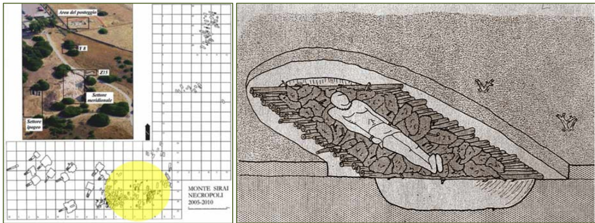
Figs. 3, 4 - El área de las necrópolis fenicio-púnicas y su extensión (GUIRGUIS 2013, fig. 28); detalle del ritual de incineración (BARTOLONI 2004, fig. 50).
