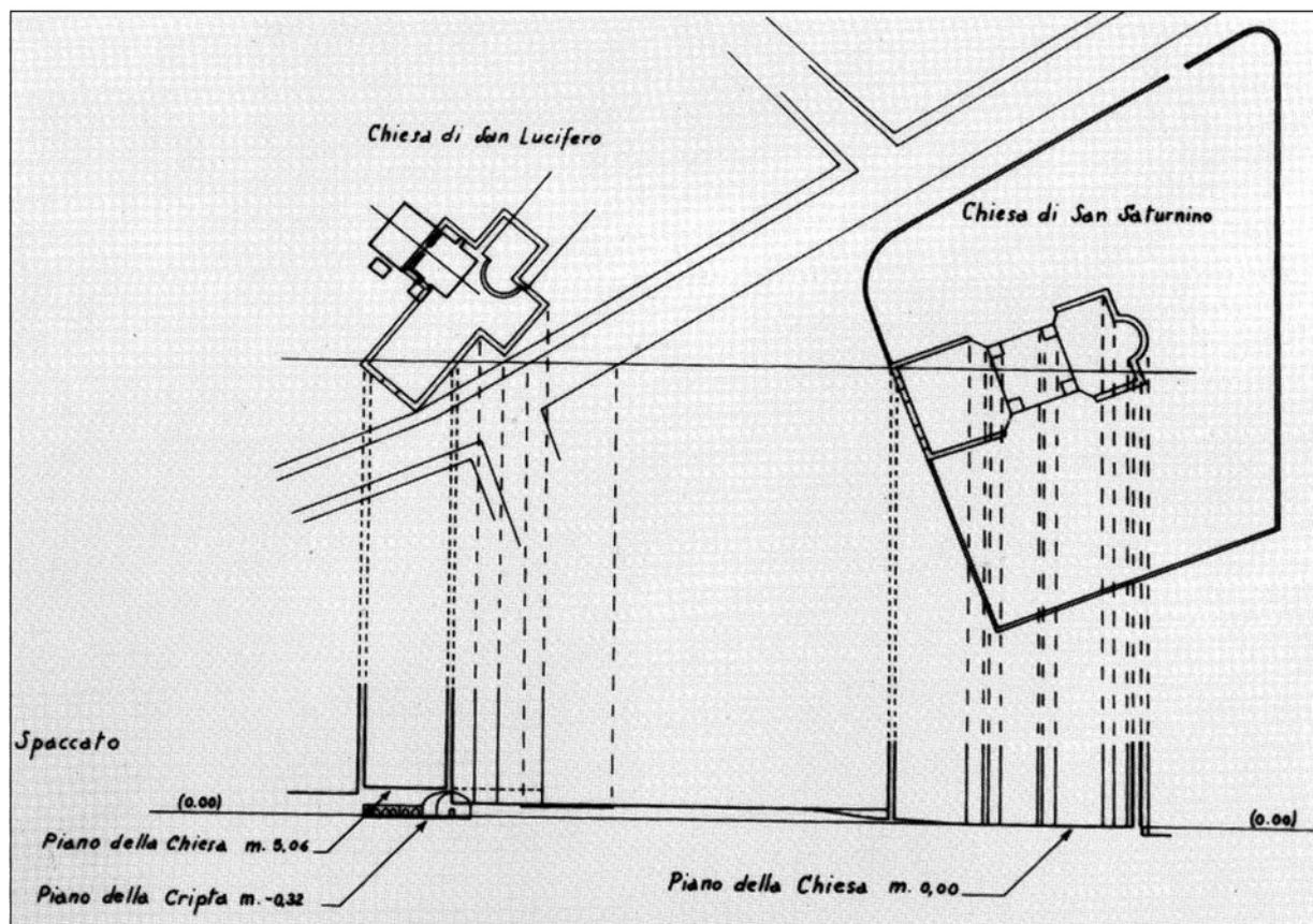
Abb. 1 - Planimetrie der Räume unter er Kirche S. Lucifero, bezogen auf die Basilika S. Saturnino (aus: Murreddu et alii 1988, S. 156, Tafel 12).
