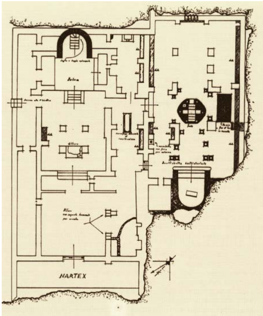
Abb. 2 - Grundriss des Episcopalkomplexes: links die Hauptbasilika (aus: FARRIS 1993, S. 100, Tafel 5).
