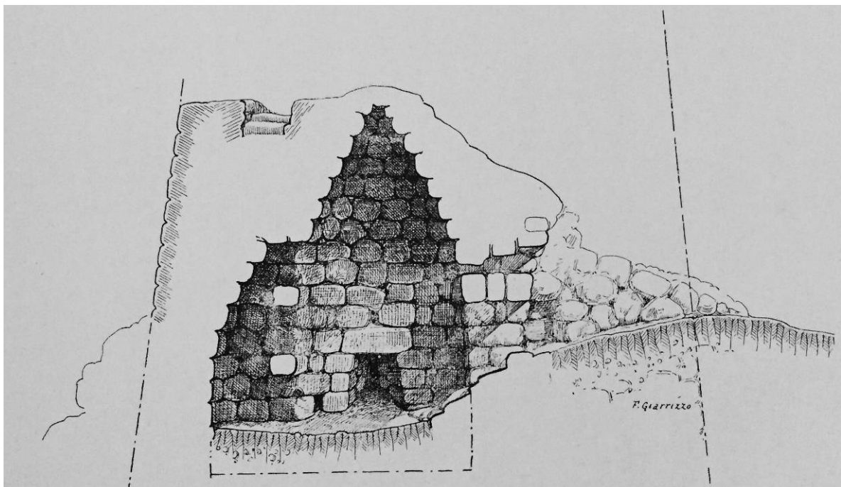
Abb. 1 - Schnitt der Nuraghe Puttu de Inza (aus: Taramelli 1919, Abb. 30, SS. 73 - 74).
