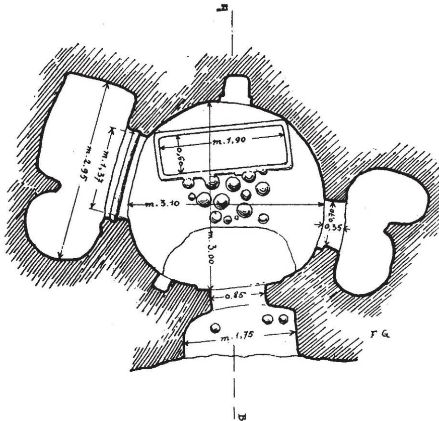
Abb. 2 - Planimetrie der domus de janas (aus: Taramelli 1919, Abb. 44, S. 102).
