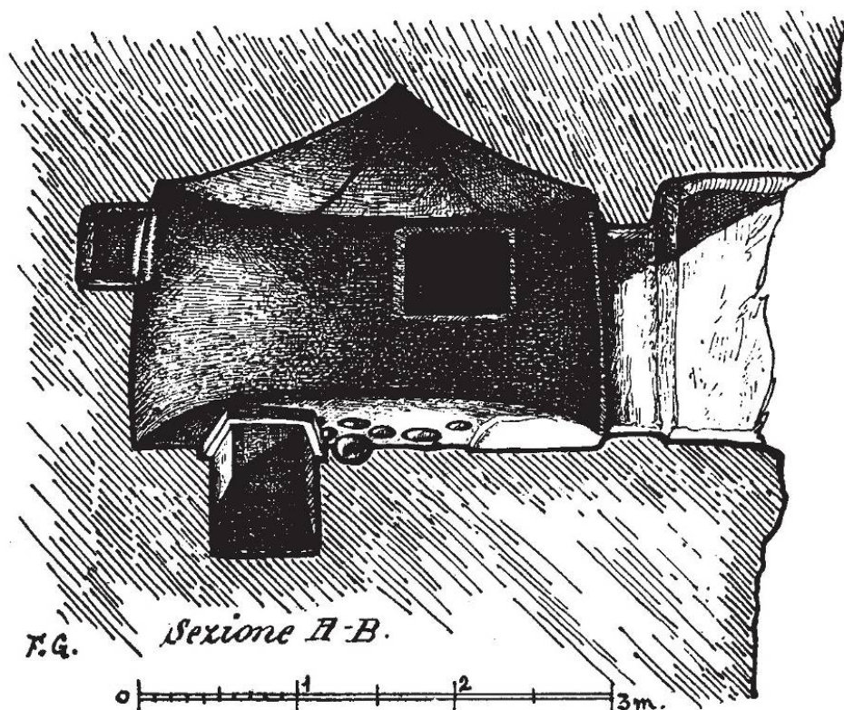
Abb. 3 - Querschnitt durch den unterirdischen Raum (aus: Taramelli 1919, Abb. 45, S. 103).
