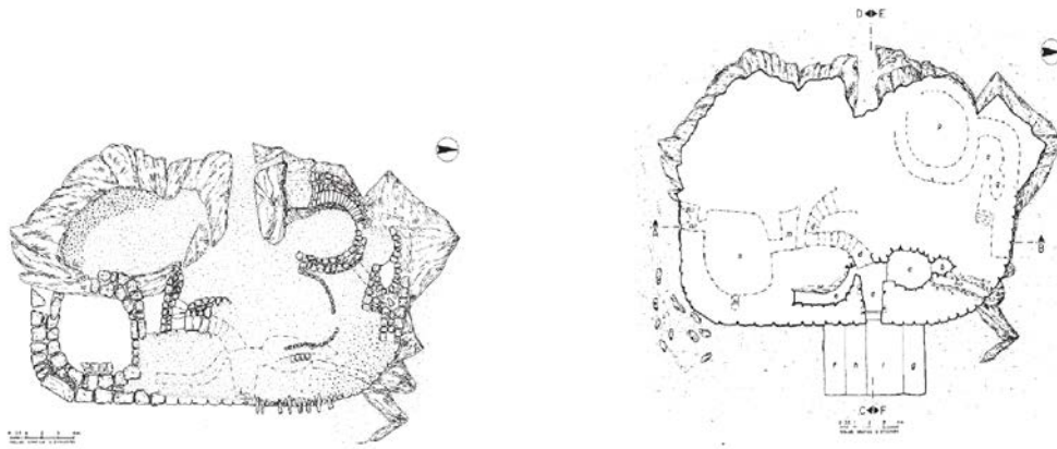
Abb. 1 - Nuraghe Albucciu, Planimetrie des Erdgeschosses und des Obergeschosses (aus: Antona Ruju, Ferrarese Ceruti 1992, Abb. 12).
