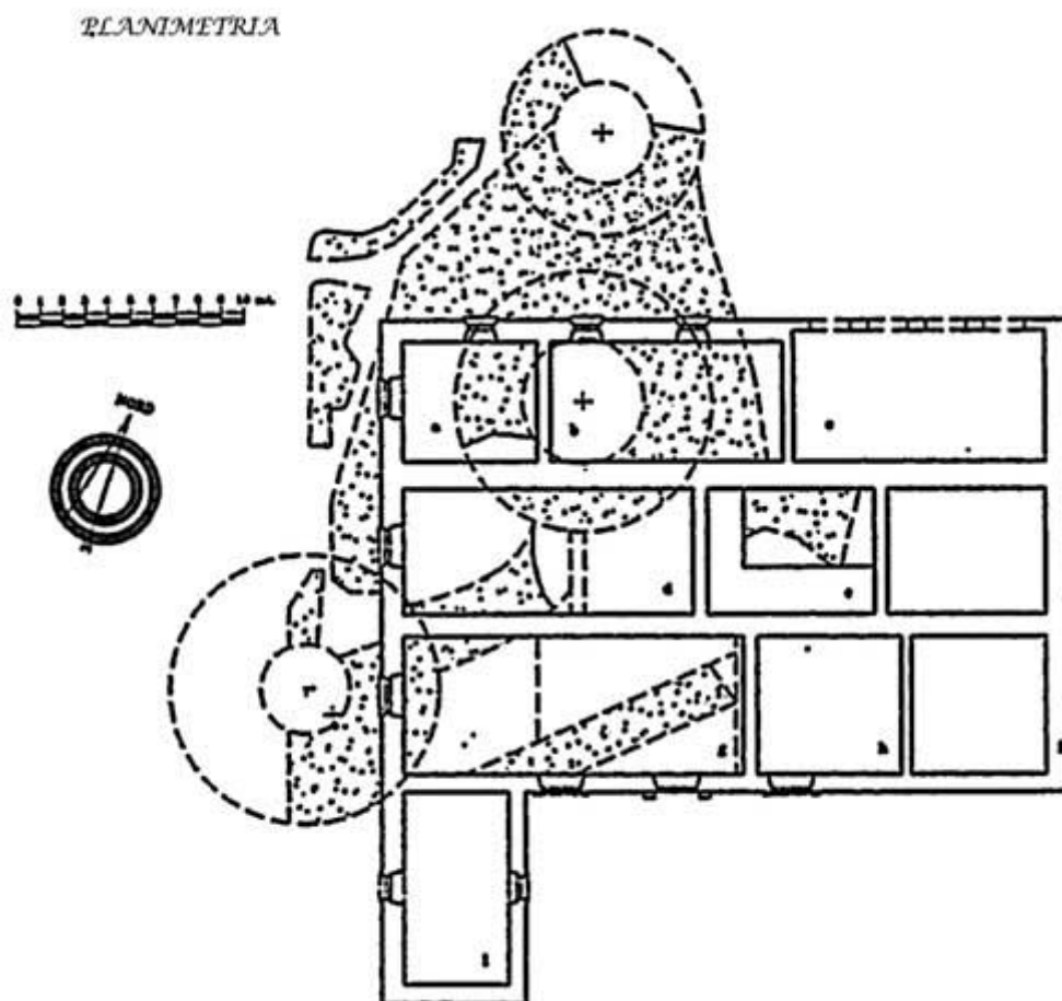
Abb. 1 - Planimetrie der archäologischen Überreste der Nuraghe Su Nuraxi 'e Cresia (von http://barumini.altervista.org/foto/planimetria-copia.jpg ).
