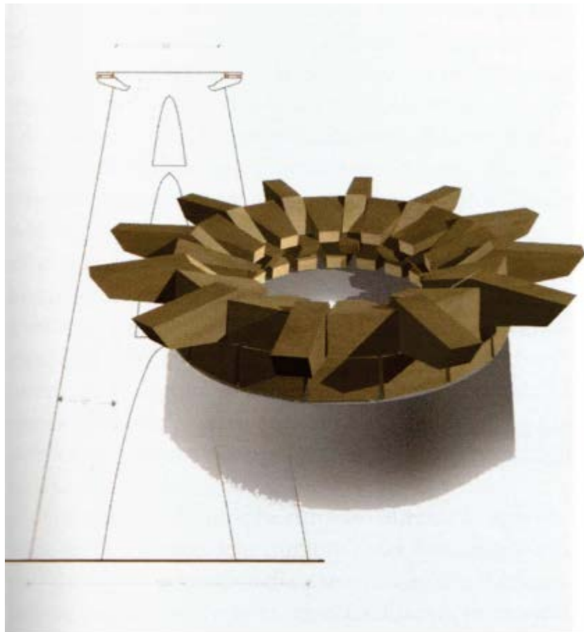
Abb. 1 - Dreidimensionale Darstellung des Systems der Terrasse des Bergfrieds von Su Nuraxi (aus: Cappai 2012, Abb. 4, S. 35).
