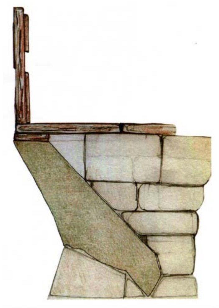
Abb. 4 - Anordnung der Simse und Keilblöcke gemäß der Rekonstruktionshypothese von Lilliu (aus: Cappai 2012, Abb. 7, S. 38).
