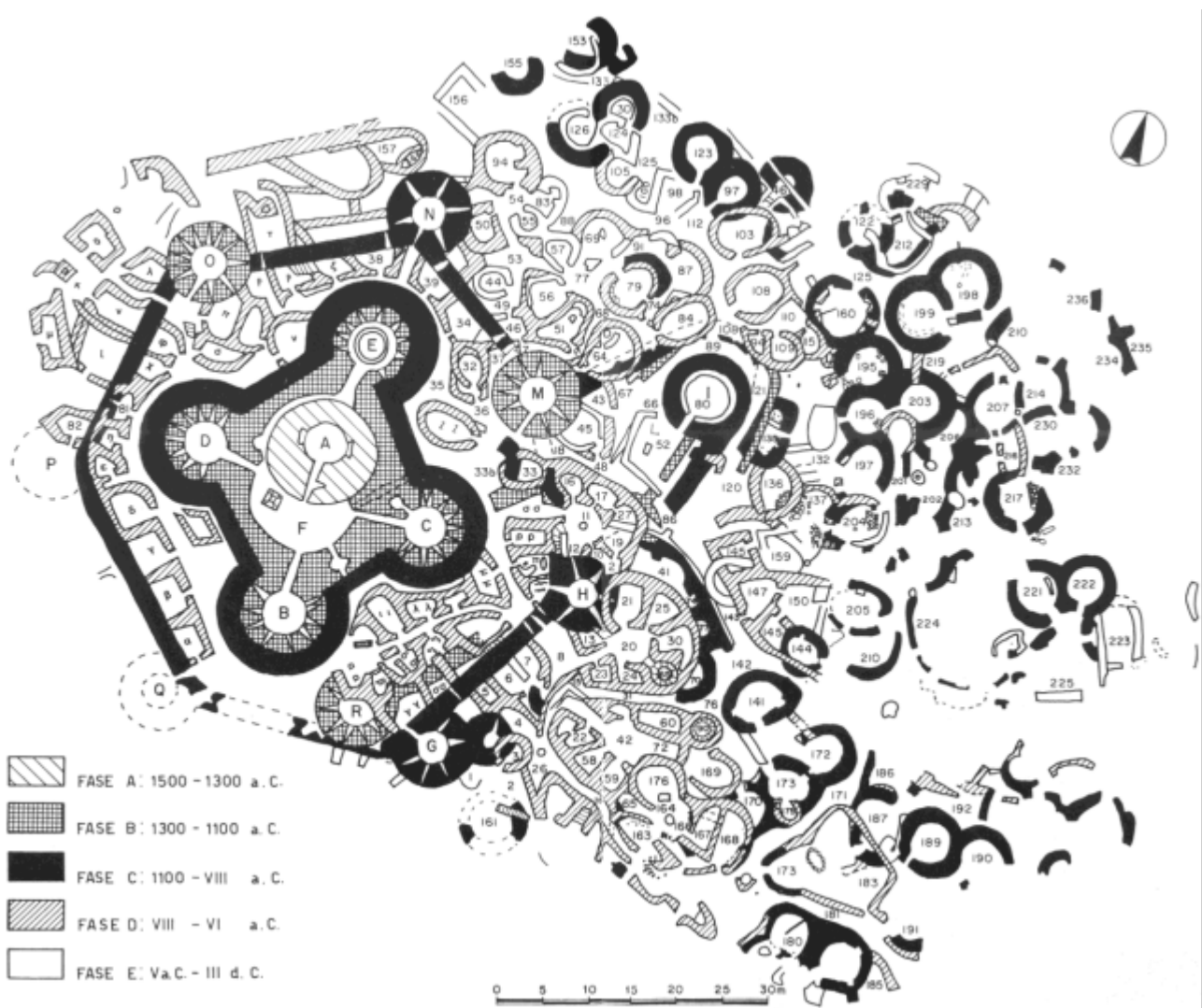
Abb. 7 - Su Nuraxi, Planimetrie des Jahres 1988 (aus: Lilliu, Zucca 1988, Abb. 25-29, SS. 48-50).
