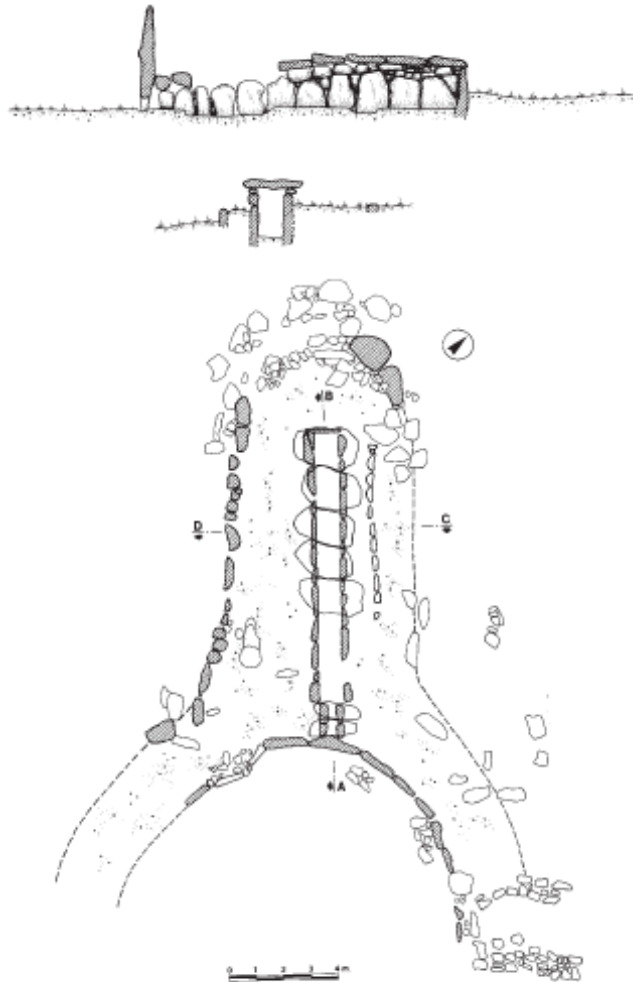
Abb. 10 - Plan und Schnitt des Gigantengrabs von Thomes (aus: Moravetti 1998, Abb. 62, S. 76).
