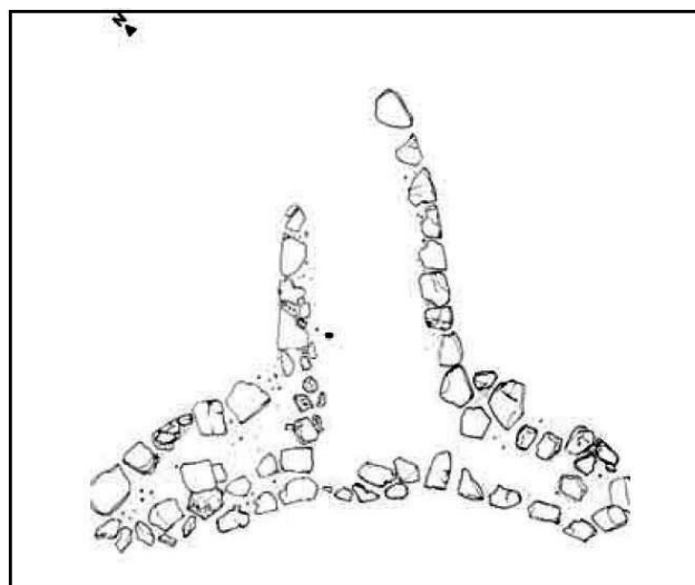
Abb. 4 - Planimetrie des Gigantengrabs von Pala Niedda (aus: FADDA 2012, S. 31, Abb. 40).
