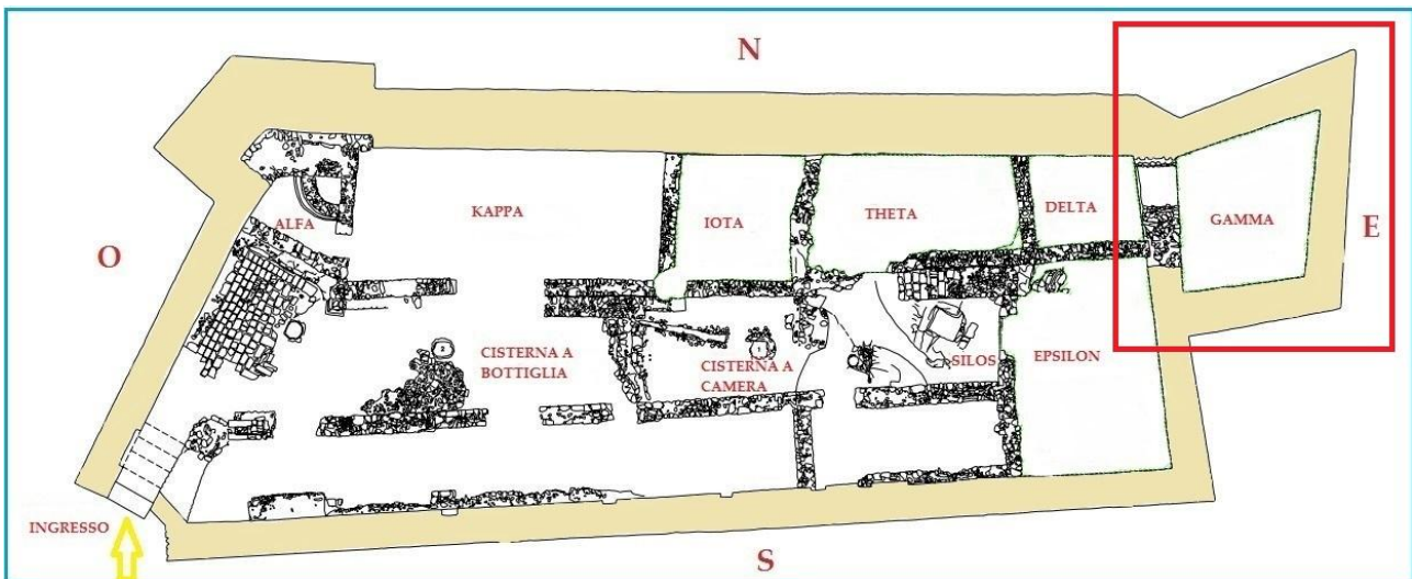
Abb. 1 - Der Raum gamma (Überarbeitung von M. G. Arru, aus: Spanu 2003, S. 58).
