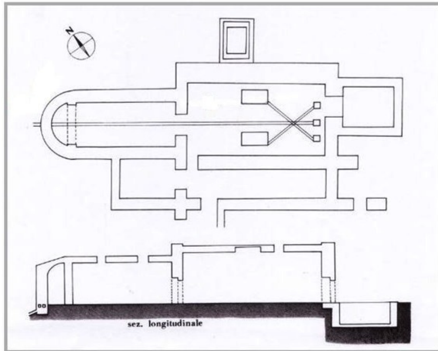
Abb. 1 - Planimetrie der römischen Thermen in der Ortschaft S. Maria de is Acquis (aus: ZUCCA 1987, Tafel 27, S. 258).
