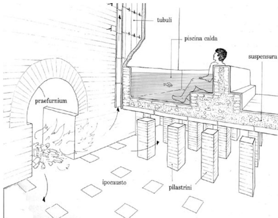
Abb. 2 - Heizungssystem der Räume: Vom Ofen gelangte die heiße Luft unter den Bodenbelag, der von Suspensurae getragen wurde, und dann durch die gelochten Tubuli im Inneren der Wände; auf diese Weise bildet sie ein warme Dämmung des Raums (aus: Adam 1988, S. 293).
