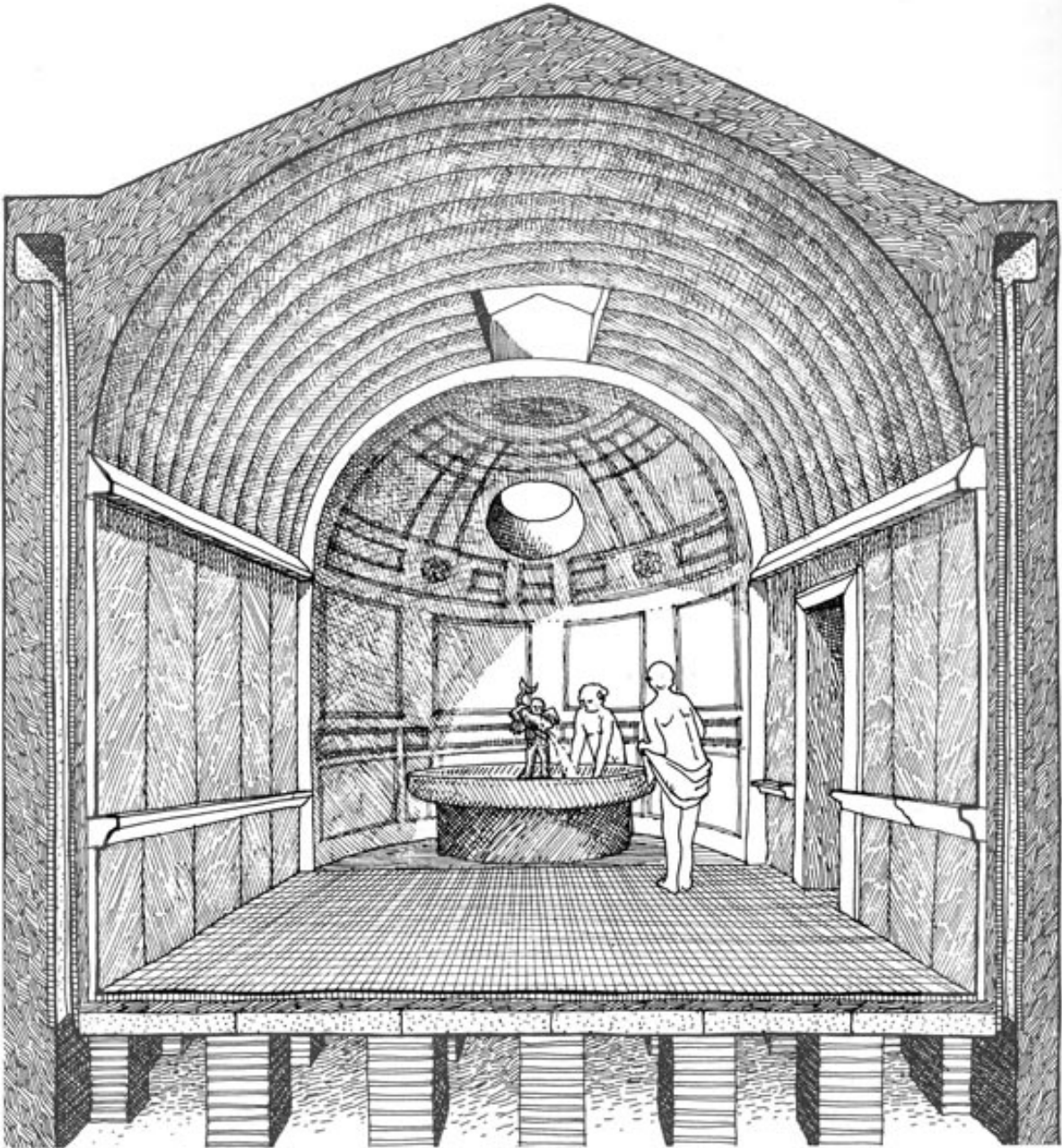
Abb. 4 - Die Rekonstruktion stellt die Apsis eines Kaldariums mit Tauchbecken zur Erfrischung dar. Zu sehen sind die Vorrichtungen für die Heizung des Raums ( Suspensurae ) sowie die Beleuchtung durch Fenster und Oberlichter (aus: Macaulay 1978, S. 86).
