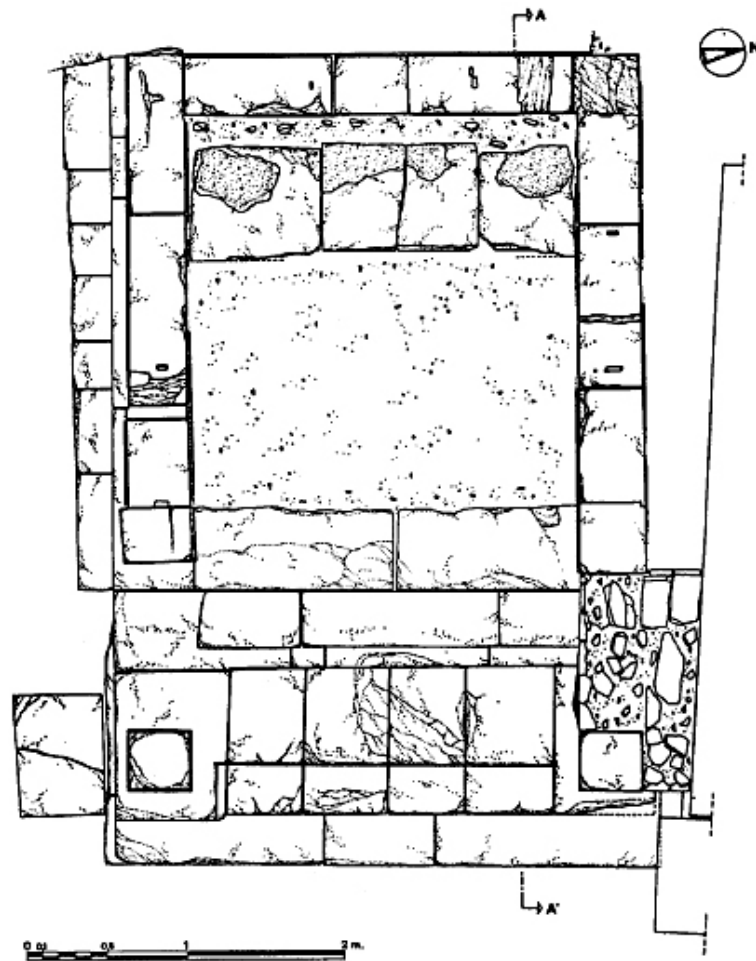
Abb. 5 - Grundriss des Tempelchens K (aus: ACQUARO 1983, S. 626)
