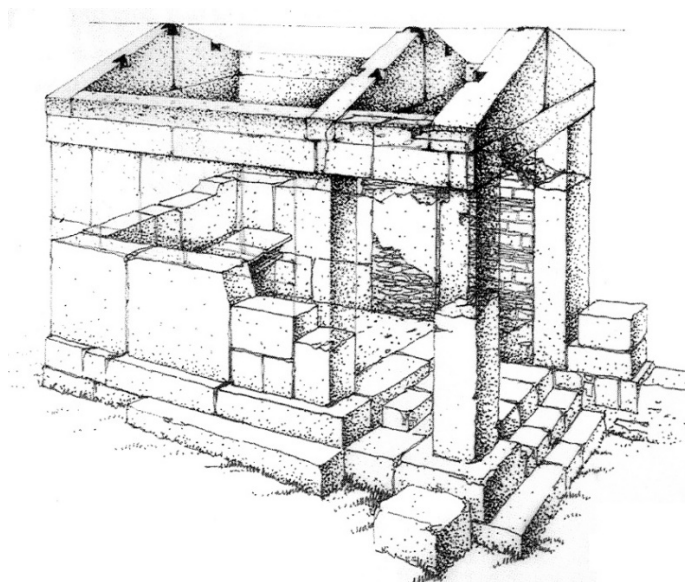
Abb. 4 - Rekonstruktion des Tempelchens K (aus: ACQUARO 1988, S. 221)
