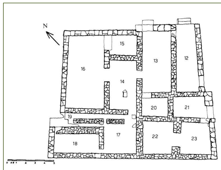
Abb. 3-4 - Das "Amadasi-Haus". Weiter oben der Astarte-Tempel; links das 'Fantar-Haus' (Foto Unicity 2015); Planimetrie (MONTE SIRAI - IV, Abb. 3).
