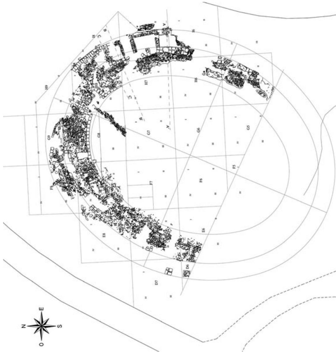
Abb. 2 - Römischer Amphitheater von Fordongianus: Planimetrie (aus Bacco et alii 2010, S. 1396).
