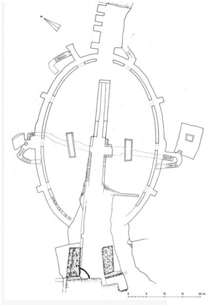
Abb. 4 - Plan des römischen Amphitheaters von Cagliari (aus: Pala 1994, S. 147).
